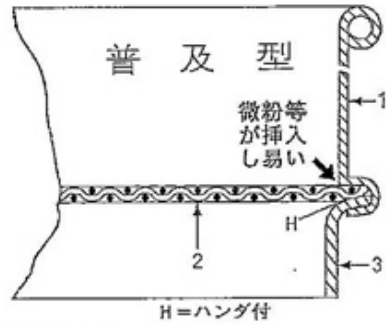
(実用新案型と普及型の構造比較断面図)
