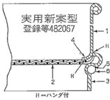
(実用新案型と普及型の構造比較断面図)
